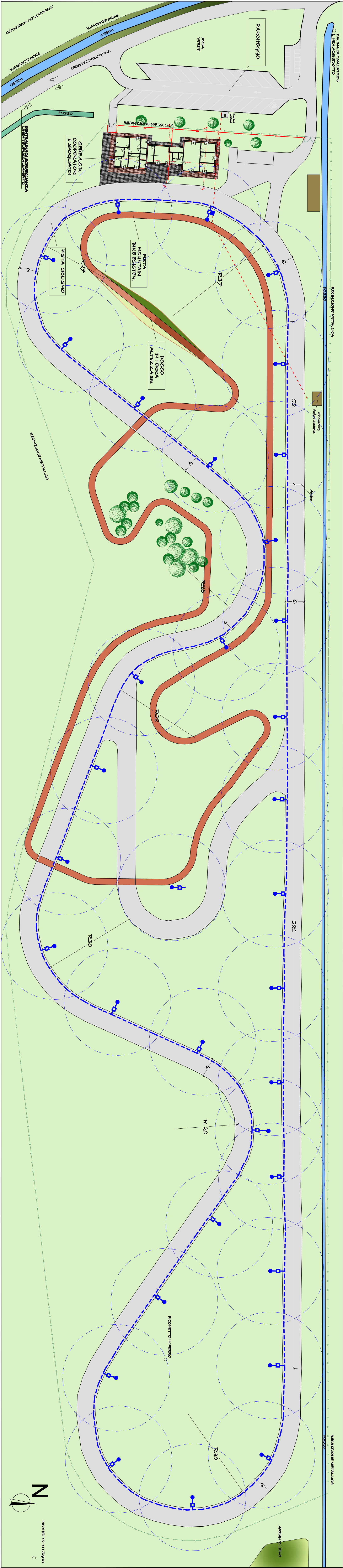
PLANIMETRIA GENERALE scala 1:500
